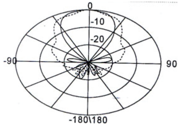
3000MHz(56° / 45° )
