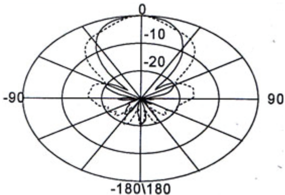
2500MHz(34° / 41° )
