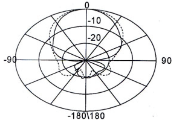
2000MHz(33° / 35° )
