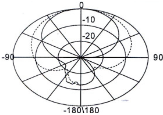
1500MHz(36° / 43° )
