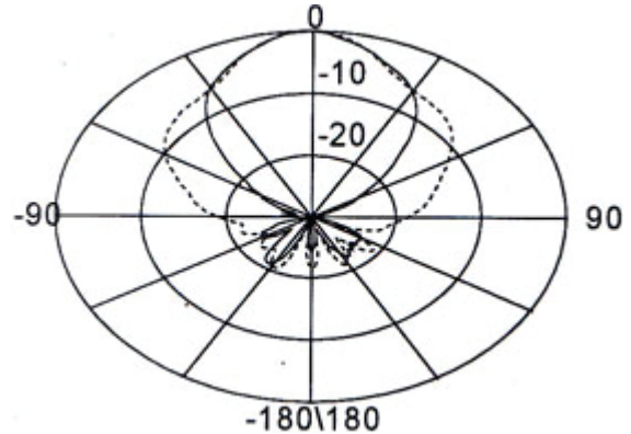
2000MHz(33° / 35° )
