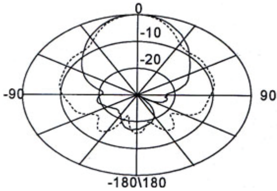
1500MHz(36° / 43° )
